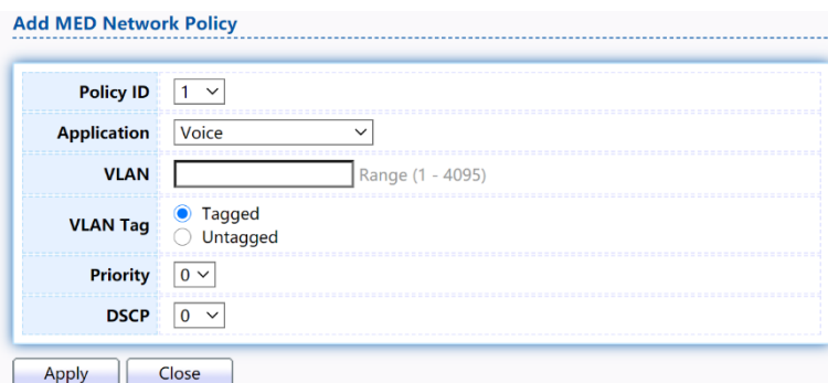
Figure 78 - Discovery > LLDP > MED Network Policy
